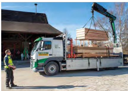
Der Kran-LKW bietet eine komfortable Möglichkeit der Zustellung auch über Zäune hinweg.
